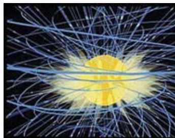
Mens solen roterer om sig selv, udslynger den plasma, der bærer på et magnetfelt, der bliver til en magnetisk spiral
